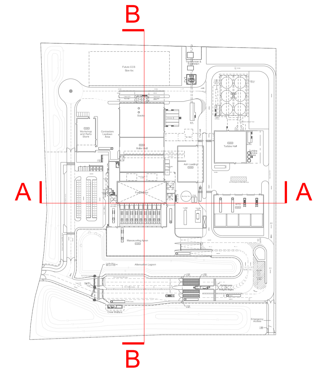
Key Plan 1:2500@A1
